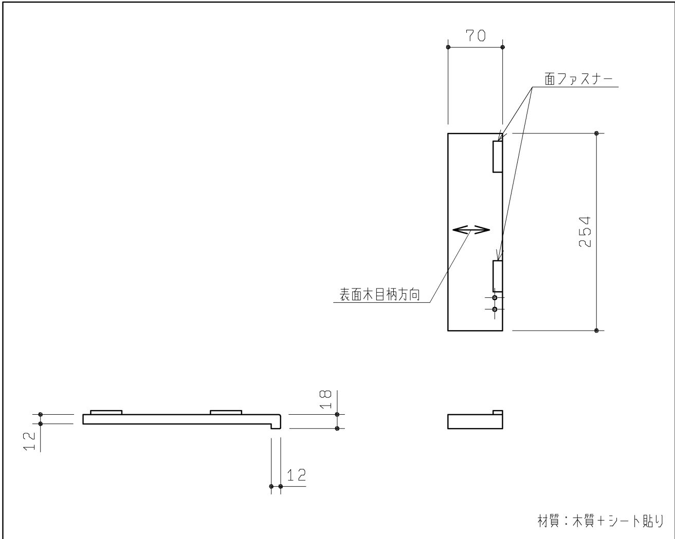
天板 ( L )
