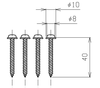
床固定ねじ
