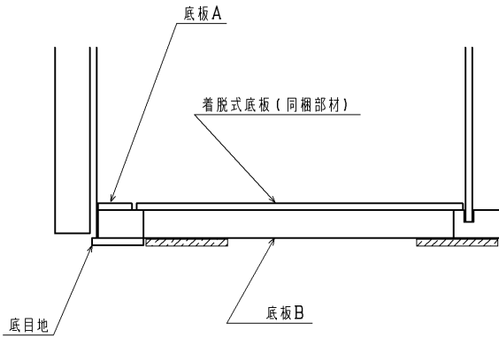
底部断面詳細図(S=1:2)
