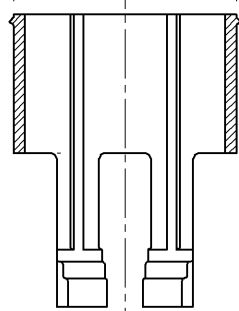
断面C-C
