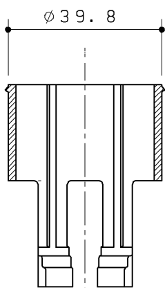
断面C-C
