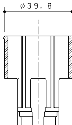
断面C-C
