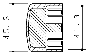
断面B-B
