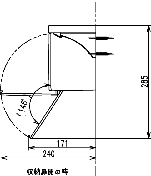
収納扉開の時
