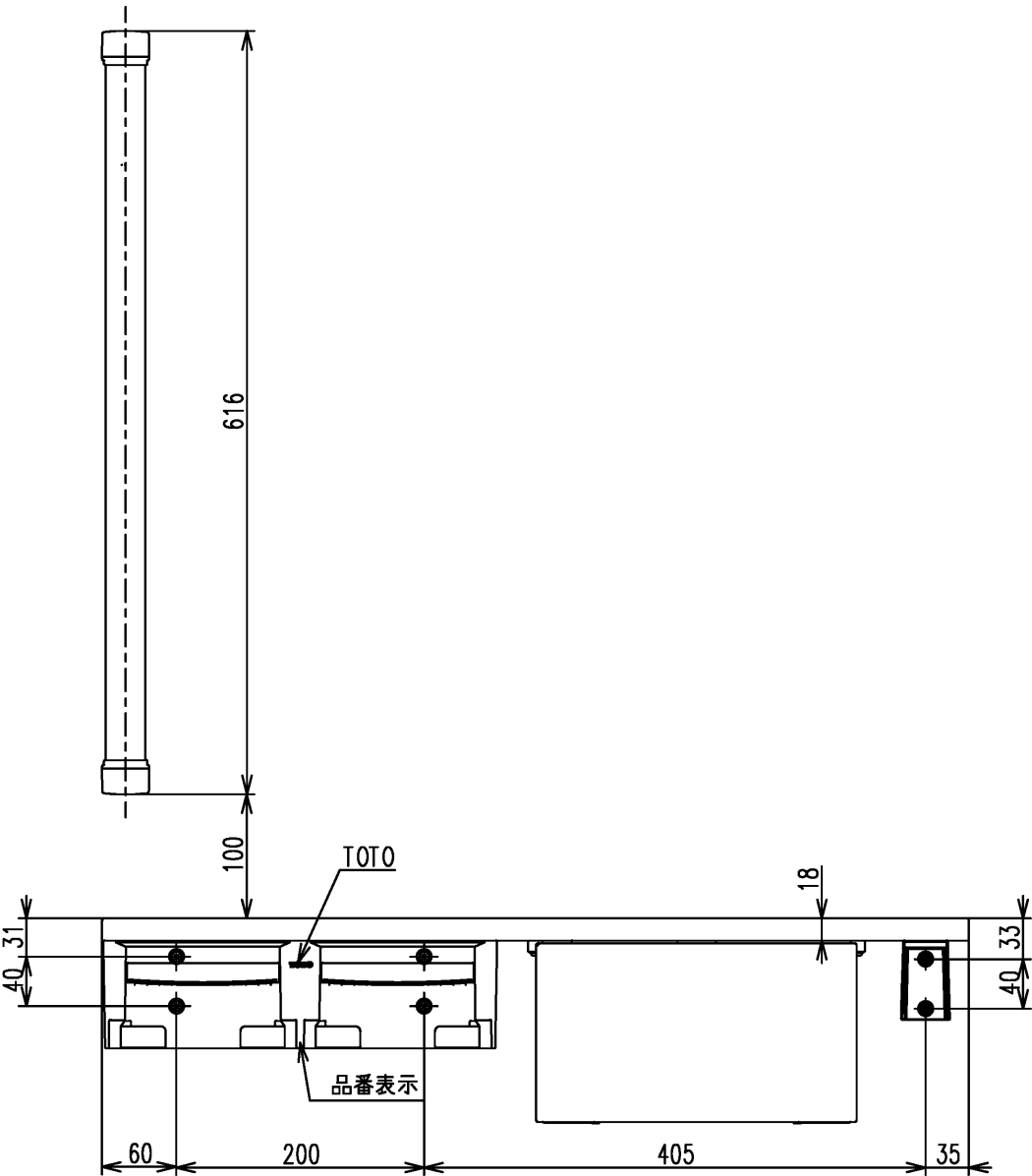
左壁設置の場合
