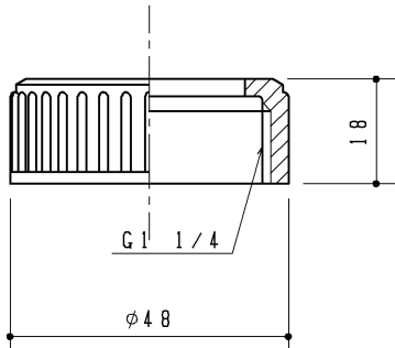
袋ナットG1（1/4）2ヶ
