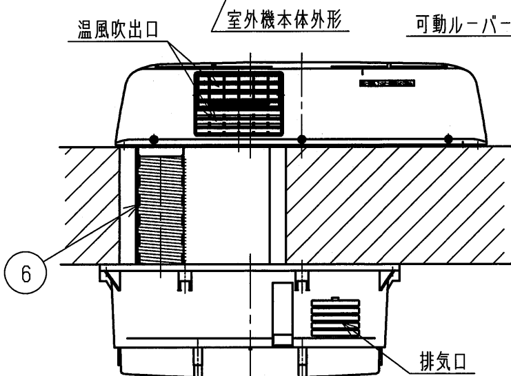
浴室ユニット（木枠内にダクトを通す場合） <右換気の時>
