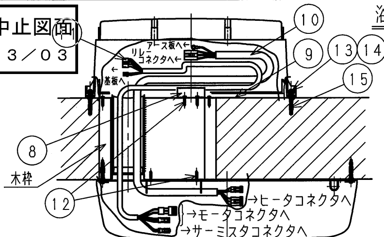
ランドリーパイプ取付位置
