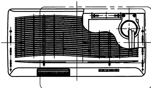
浴室ユニット（木枠内にダクトを通す場合） <右換気の時>
