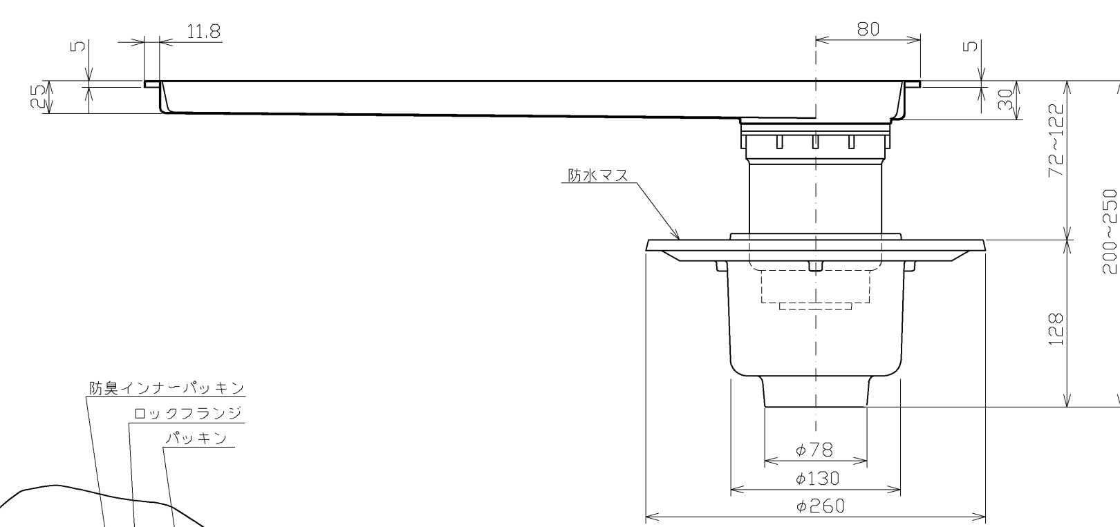
A-A' 断面 (排水ユニット本体)
