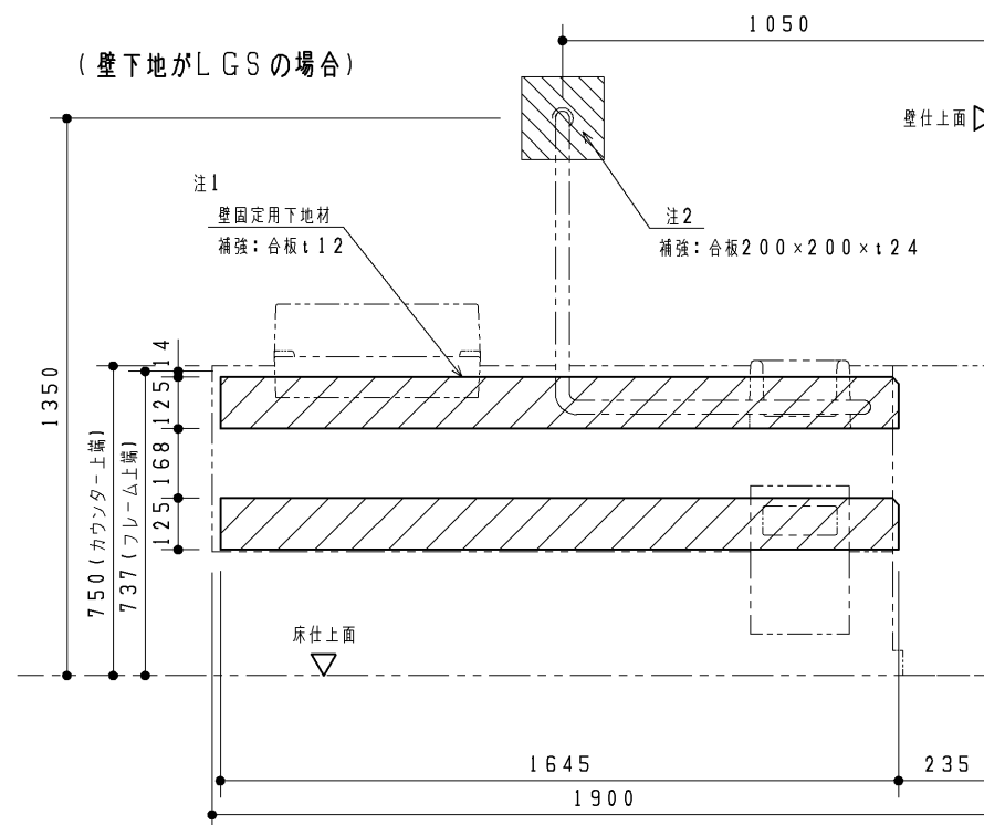
壁ハンガー部詳細 (S = 1 : 4) フレーム上端 壁固定部×3ヶ所 136 (壁ハンガー下底) 151 51 51 20 12
