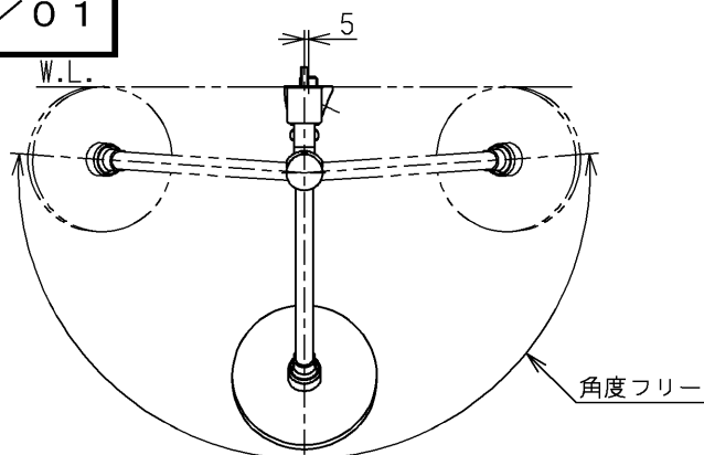
サーモ取付脚部詳細 (1:5)
