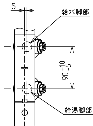
サーモ取付脚部詳細 (1:5)
