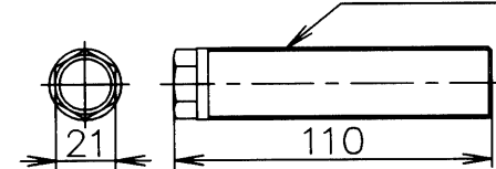
■ステーパイプB
