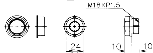
■ステーパイプA
