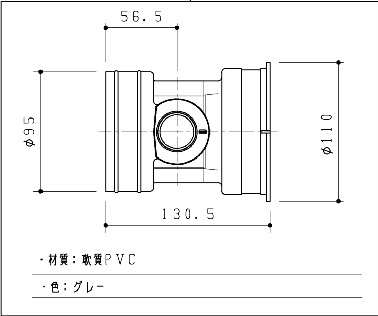
壁排水ゴムジョイント本体
