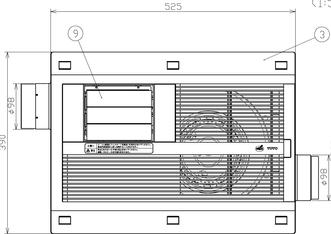
天井取付図 (1:5)
