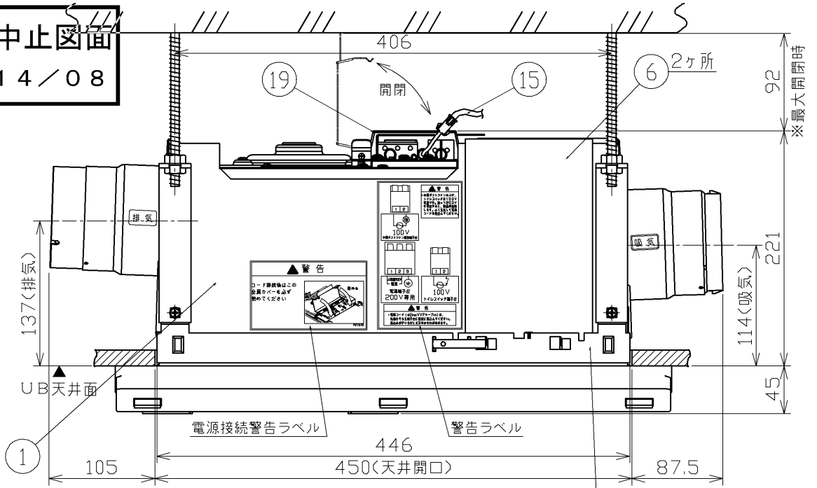
天井取付図 (1:5)
