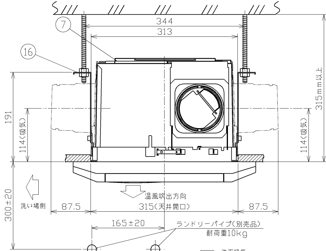
天井取付図 (1:5)
