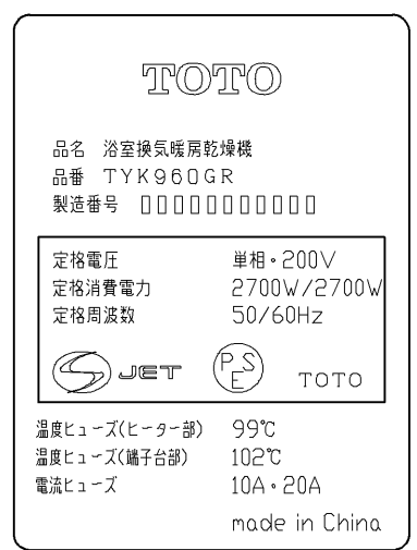
⑧ 製品銘板
