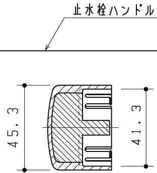
断面B-B
