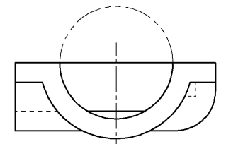
防露カバー（二方分岐用ふた）
