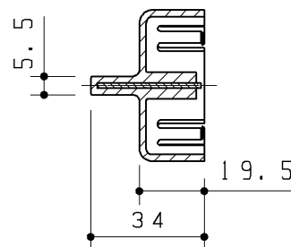
断面A-A
