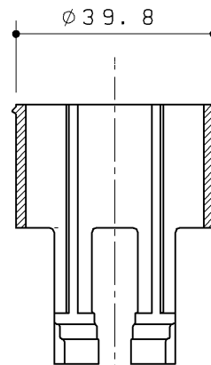
断面C-C
