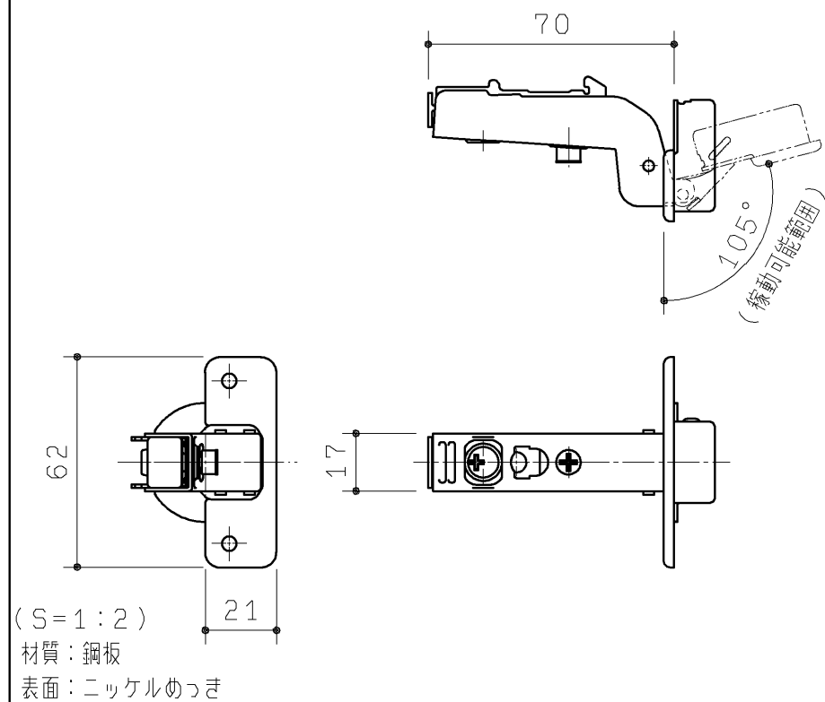
ワンタッチスライド丁番(2ヶ)
