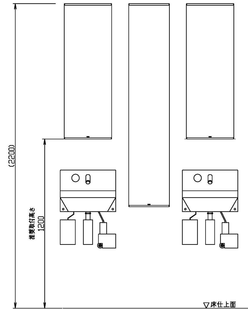
全身鏡・化粧鏡を併設したプランの取付高さ推奨取付位置
