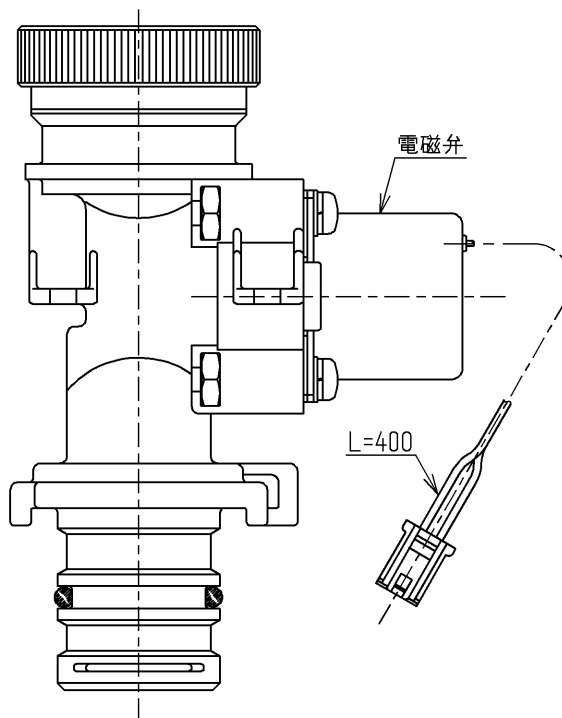
駆動部 (2個)
