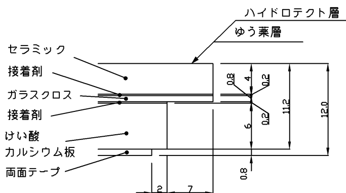
A部（断面図）拡大図2：1
