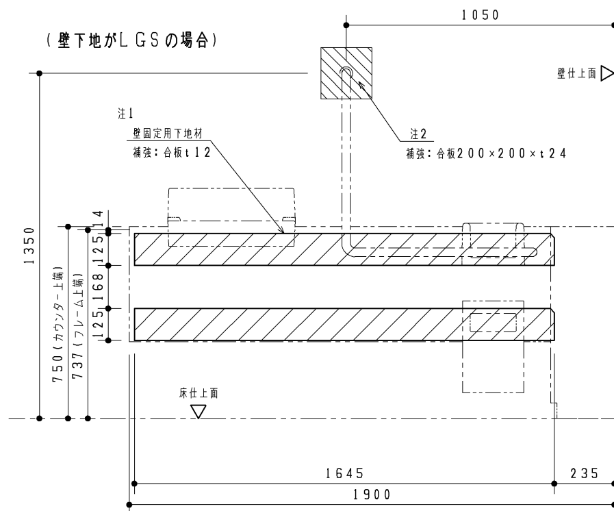
壁ハンガー部詳細 (S = 1 : 4) フレーム上端 136 ( 壁ハンガー下縁 ) 壁固定部×3ヶ所 20 12 15 15 15
