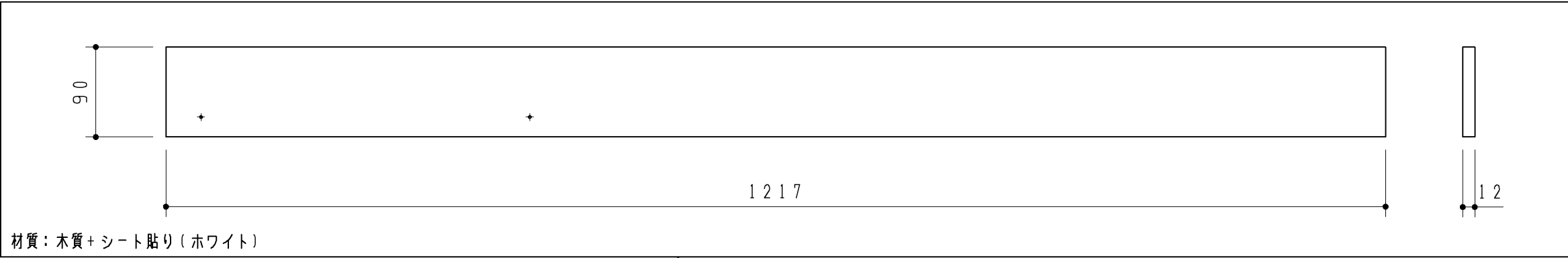
上段補強板
