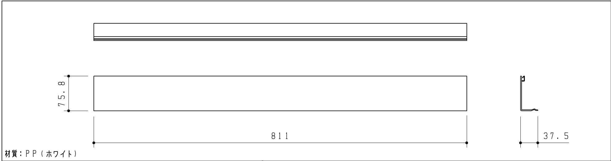
配管カバー
