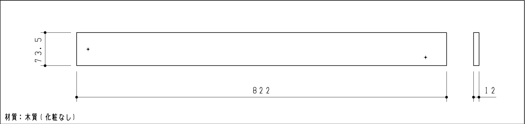
下段補強板
