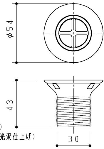
排水金具
