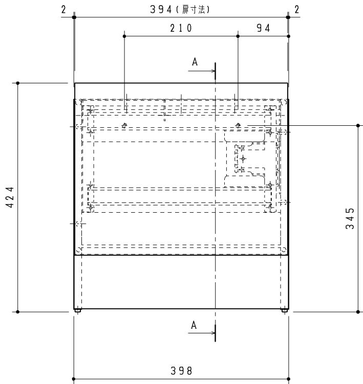
サイドキャビネット (ハーフ) 扉Rセット
