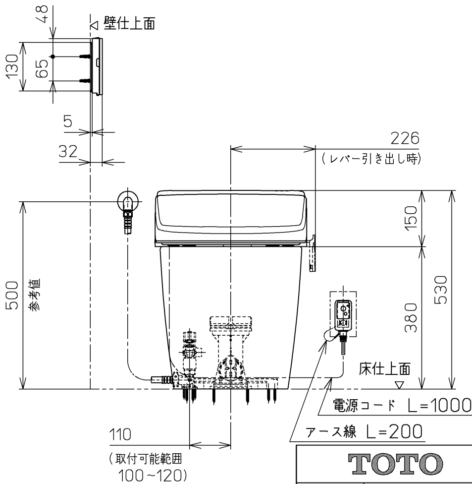
壁給水仕様の場合
