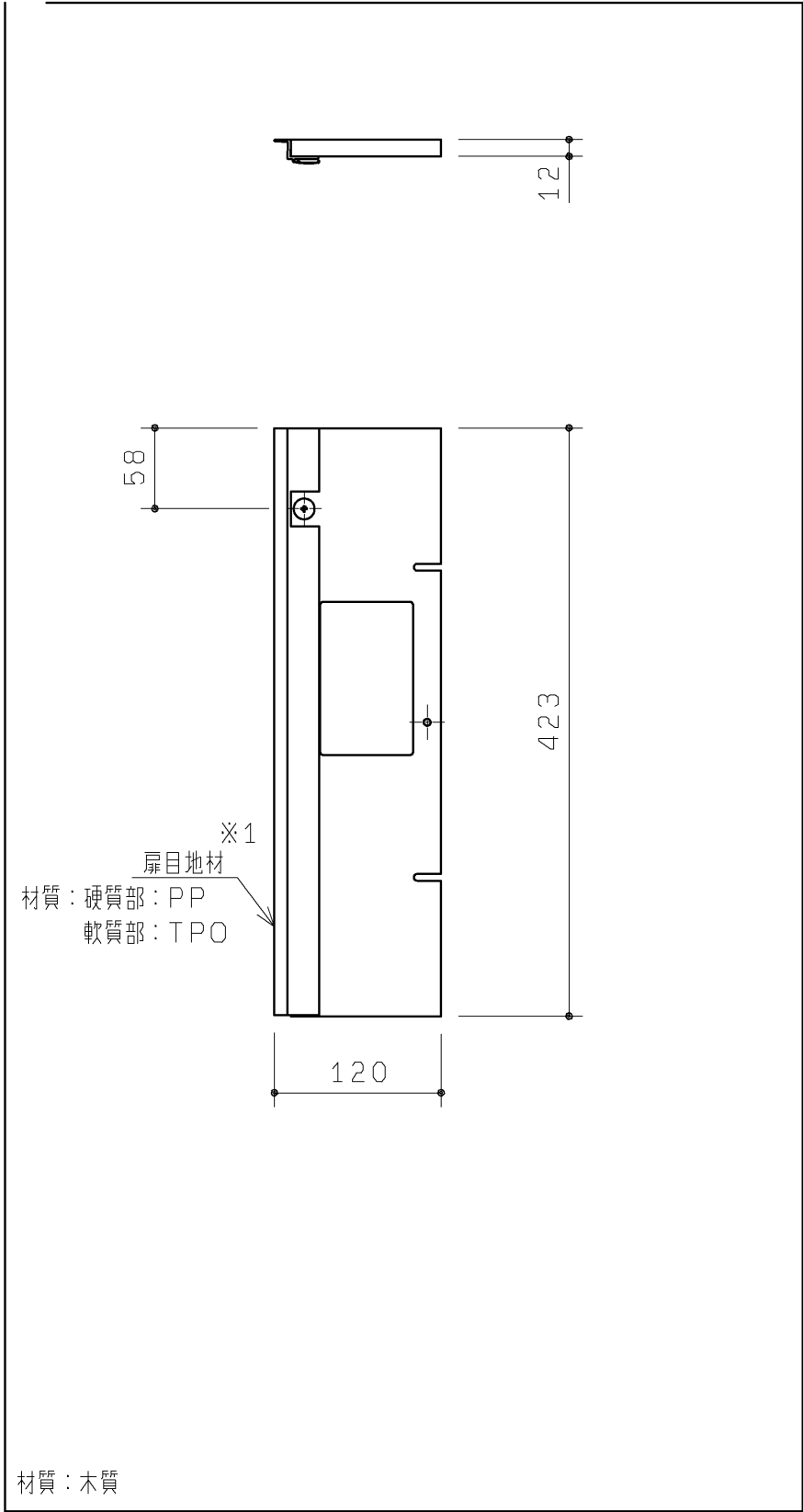
裏扉セット
