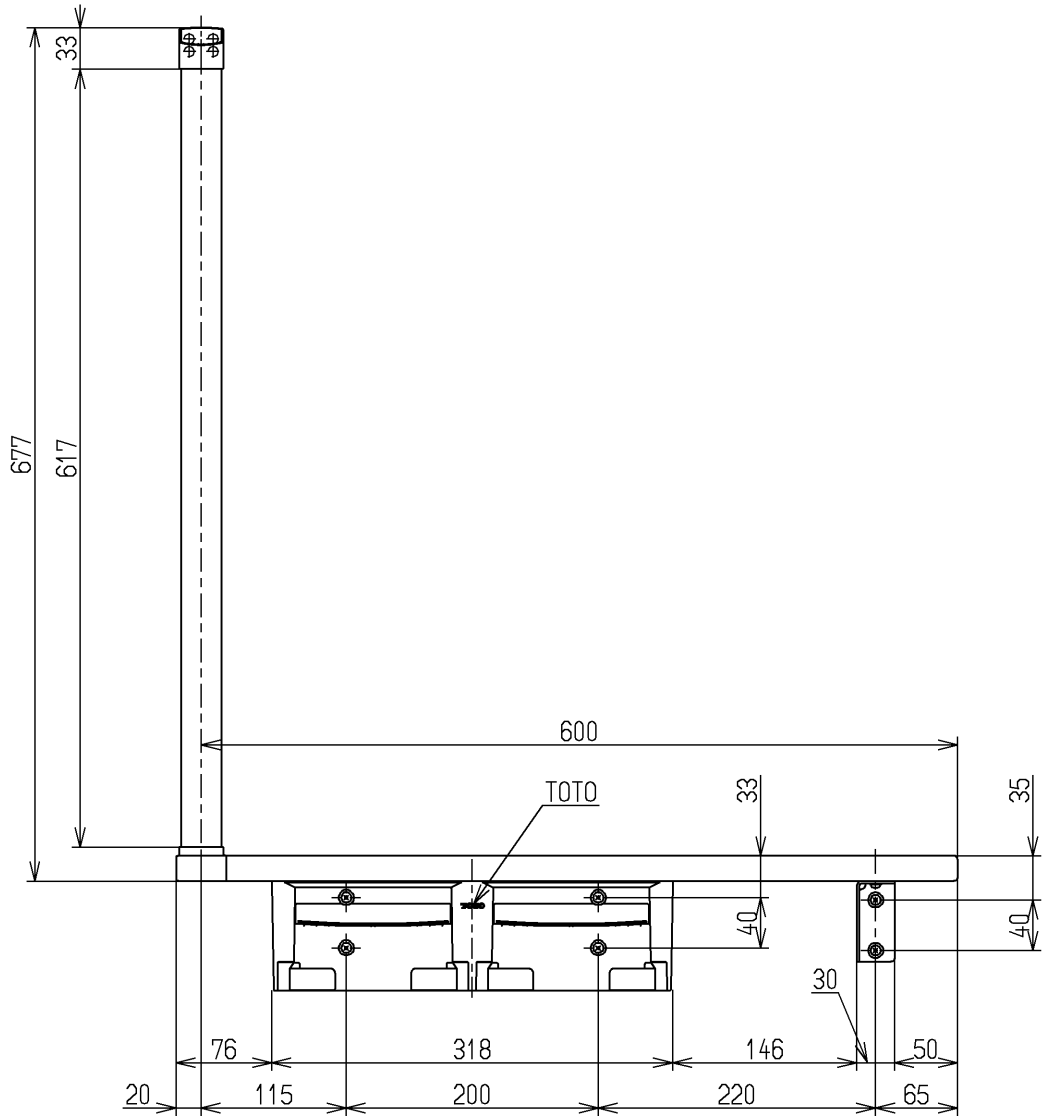
左壁設置の場合
