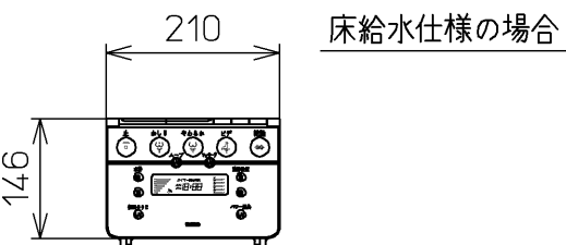
正面図
