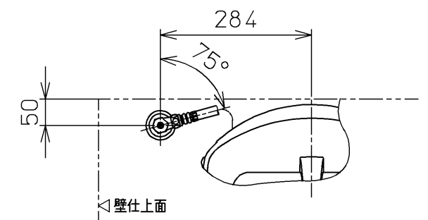
平面图
