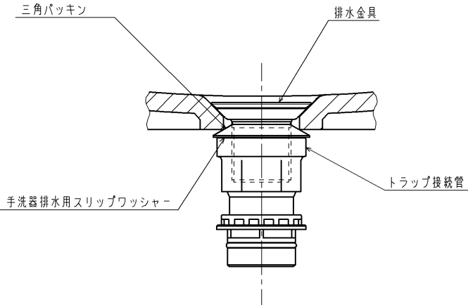
A-A (S=1:2)
