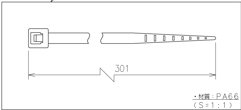
結束バンド
