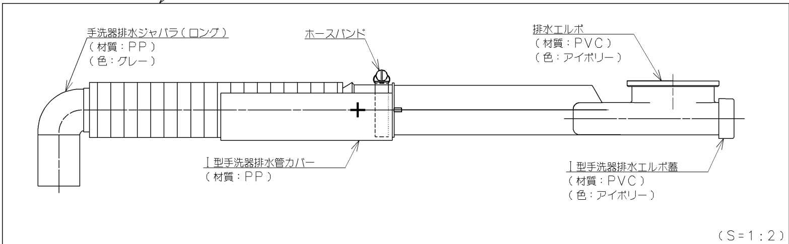
接続管組品
