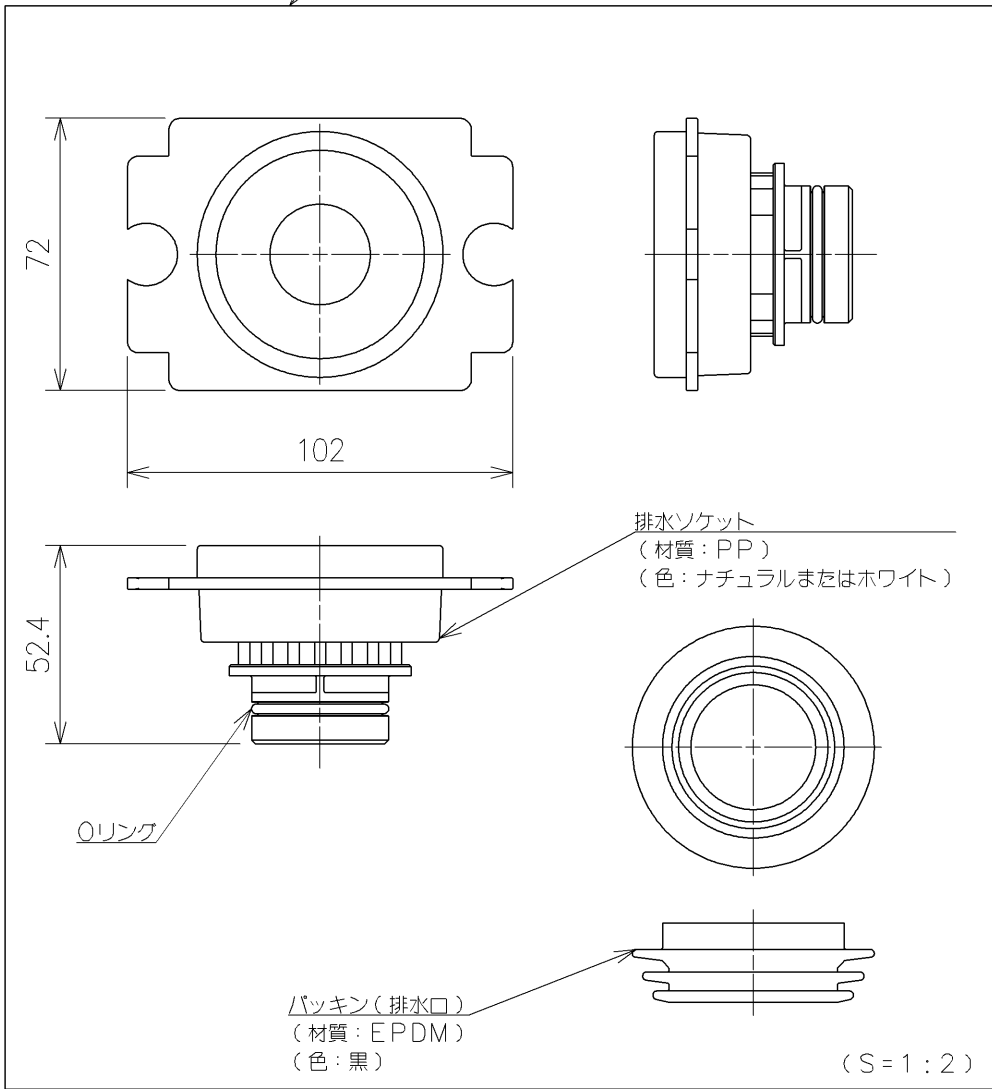
排水ソケット組品
