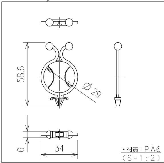
ケーブルクリップ
