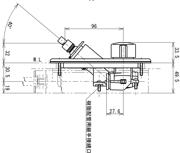
※1部詳細図（1：1）
