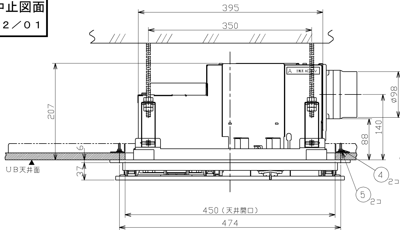
天井取付図
