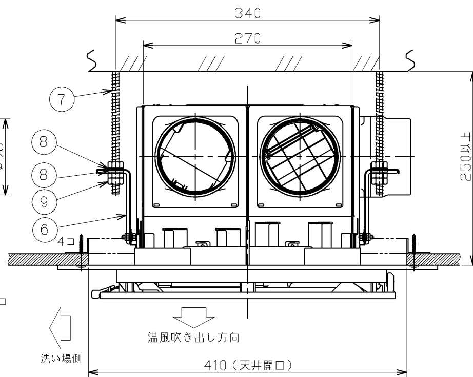
天井取付図
