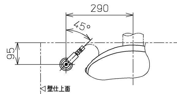
平面図
