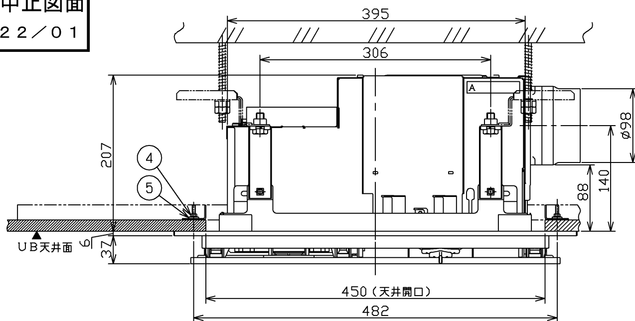
天井取付図
