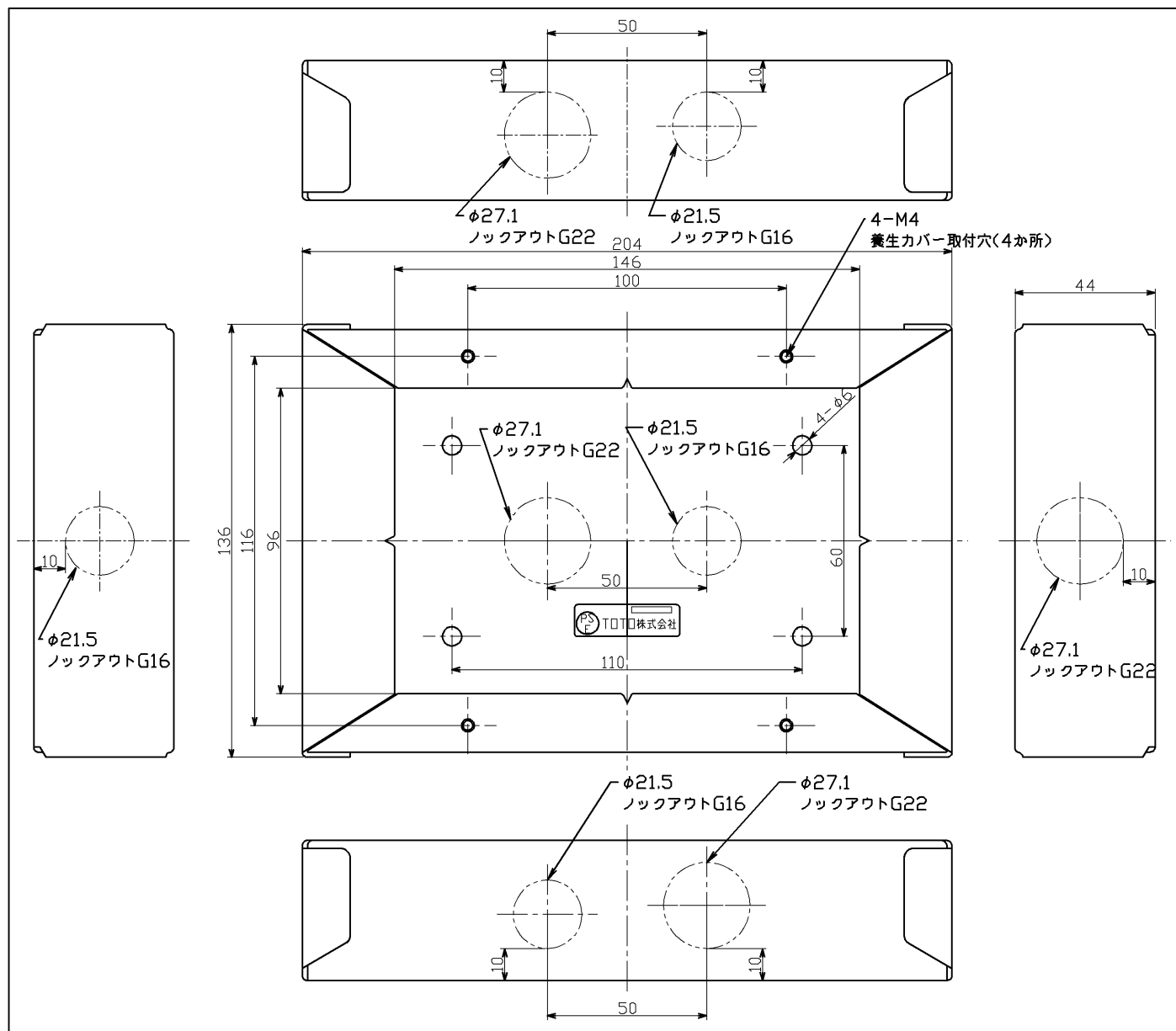
埋込ボックス（鋼板製 t=1.6 ）
