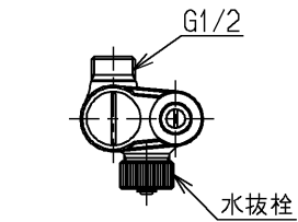
止水栓部(2ヶ)
