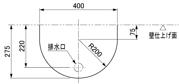
カウンター切込寸法
