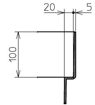
壁のせ部 (防水リム部) 詳細
