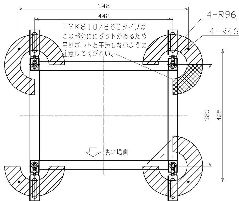
アンカーボルト取付位置TYK800タイプ(フリー)
