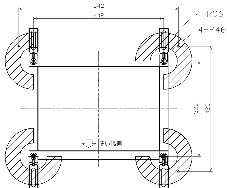
アンカーボルト取付位置 TYK150タイプ(フリー)
