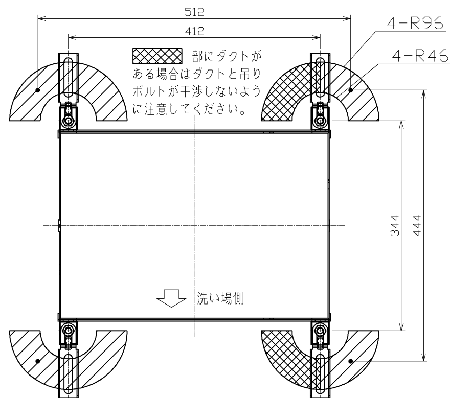
アンカーボルト取付位置TYK900タイプ(フリー)
