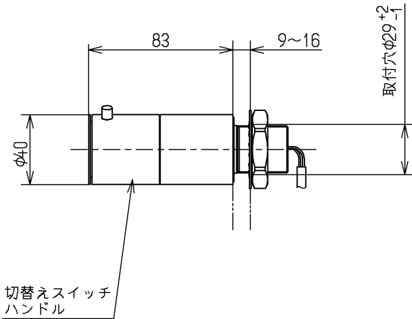
湯水切替スイッチ
