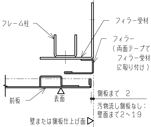
前板端部納まり詳細図（S＝1：2）
