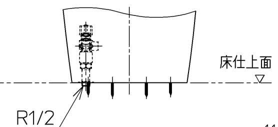
正面図 床給水仕様の場合
