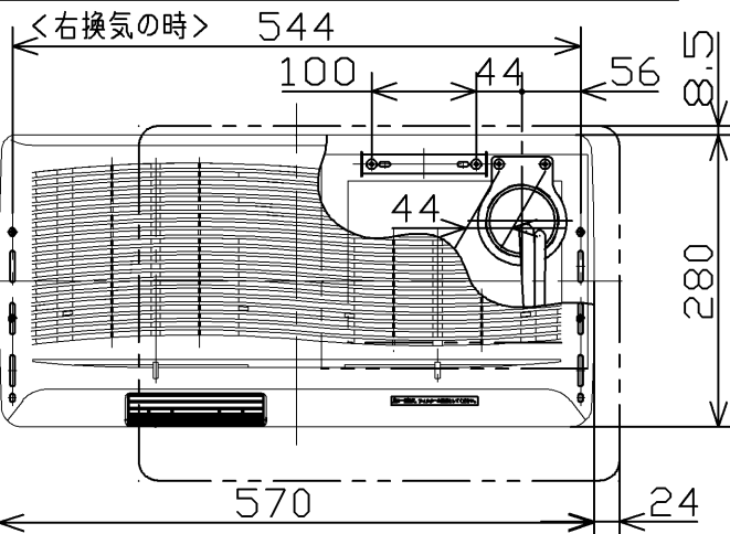
浴室ユニット（木枠内にダクトを通す場合）
