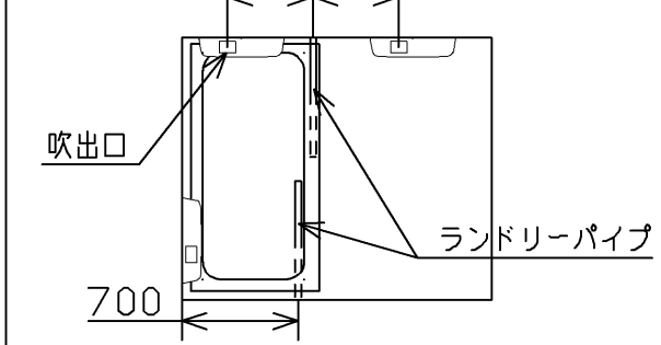
ランドリーパイプ取付位置
