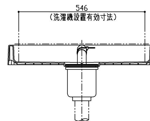
断面B-B
