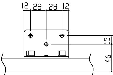
壁固定位置詳細（1/10）
