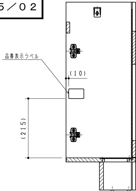
ラベル貼付位置 手洗器用キャビネット本体WLセット
