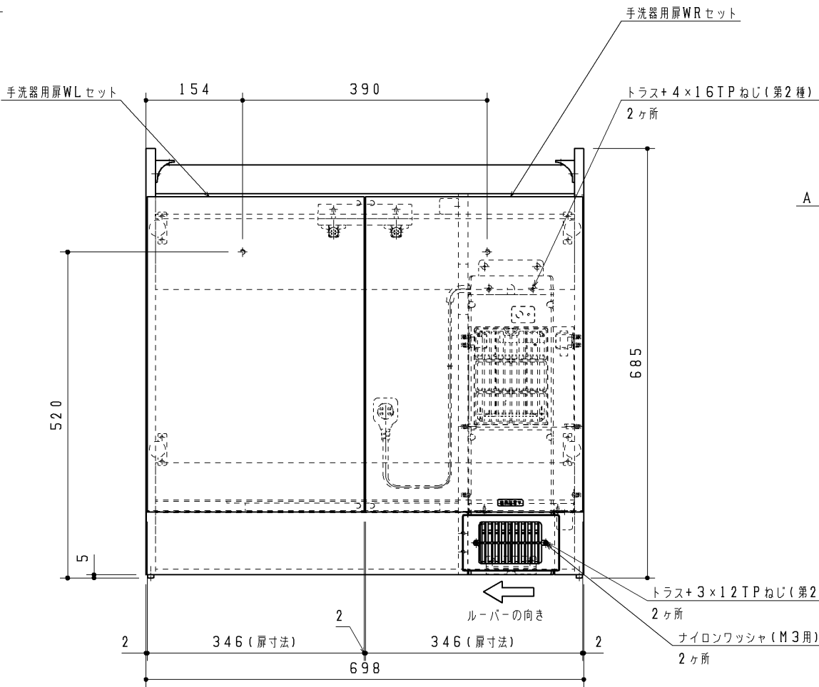
ラベル貼付位置 手洗器用キャビネット本体WLセット
