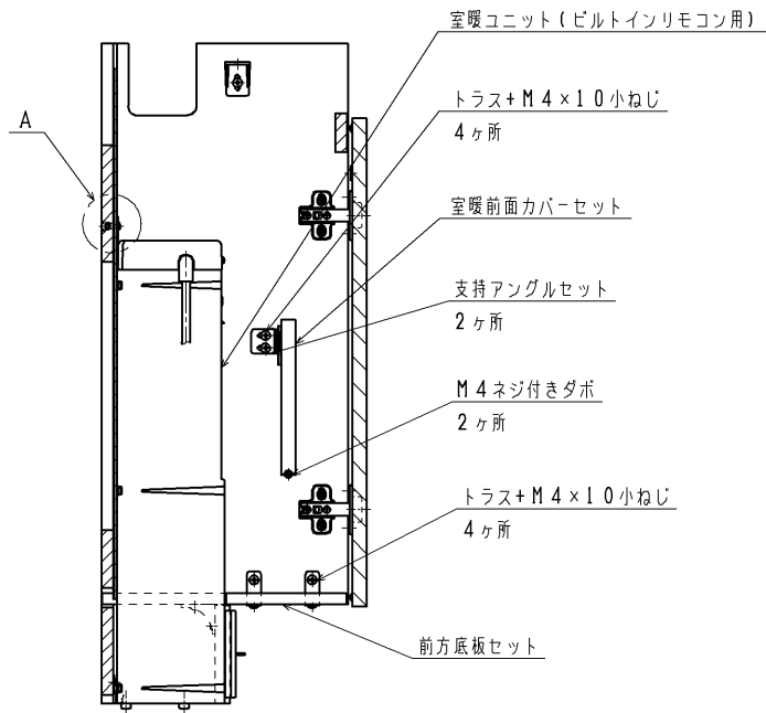
室暖ユニット固定詳細
