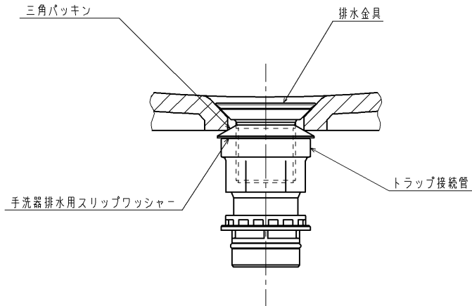
A-A (S=1:2)
