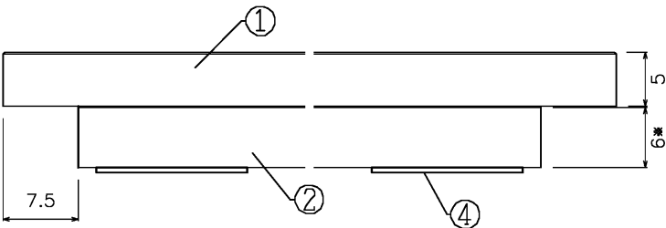
B-B断面図
