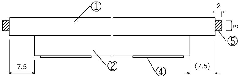
A-A断面図
