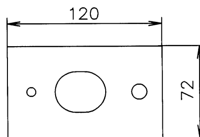
■取付板パッキン
