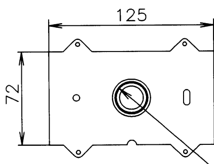
■取付板
