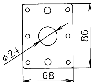
■カセットパッキン
