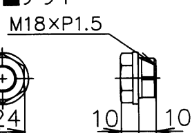
■ナット
