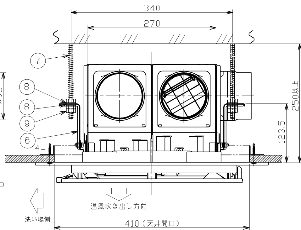
天井取付図
